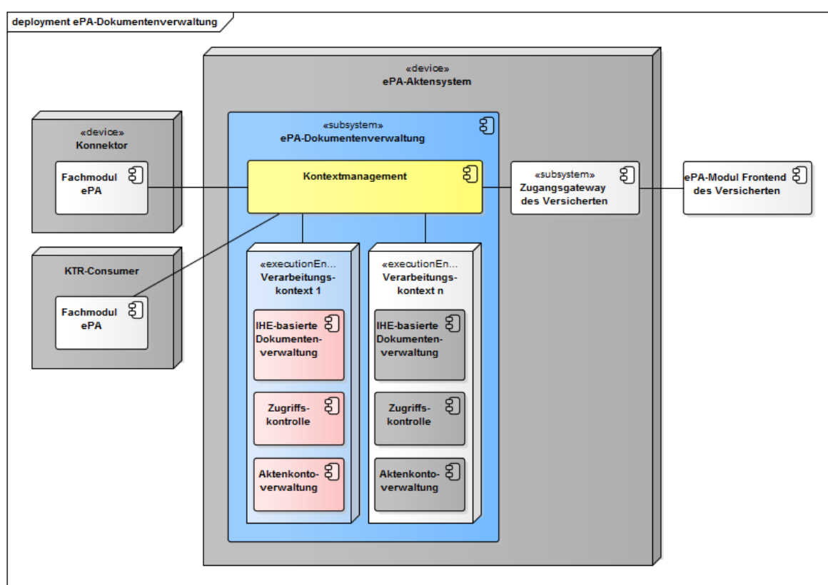
Abbildung 1: Komponentenzersetzung ePA-Dokumentenverwaltung
