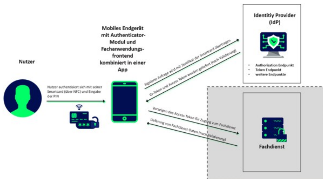
Abbildung 3: Systemüberblick (vereinfacht)
