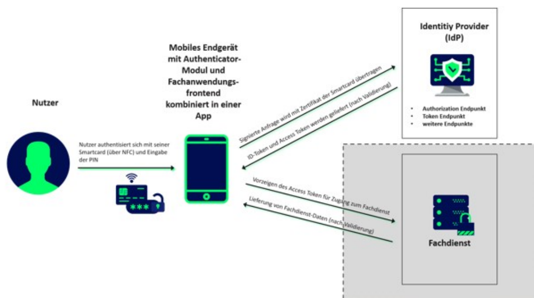
Abbildung 3: Systemüberblick (vereinfacht)
