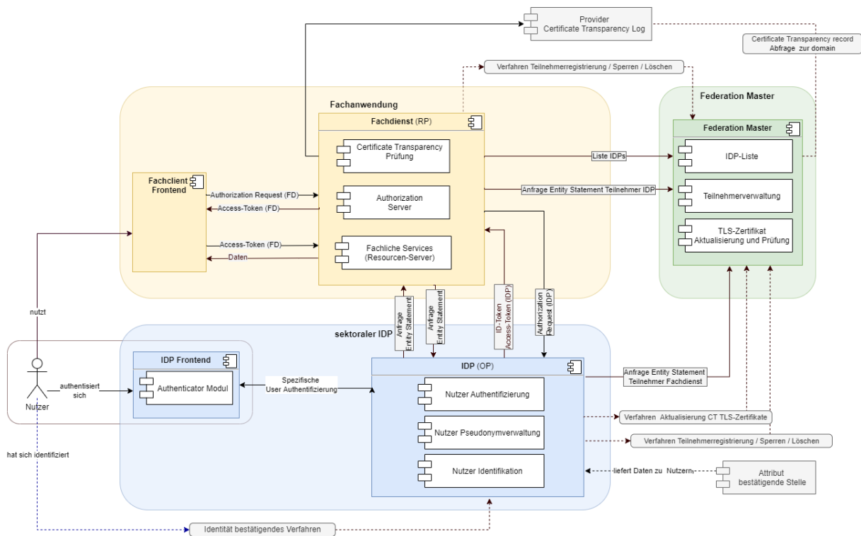
Abbildung 2: Systemkontext
