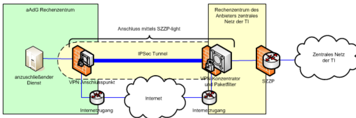
Abbildung 8: Abb_zentrNetz_SZZP-light
