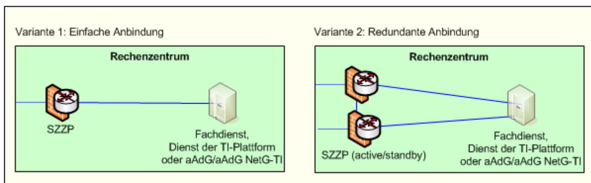
Abbildung 7: Abb_ZentrNetz_Anbindungsvarianten SZZP
