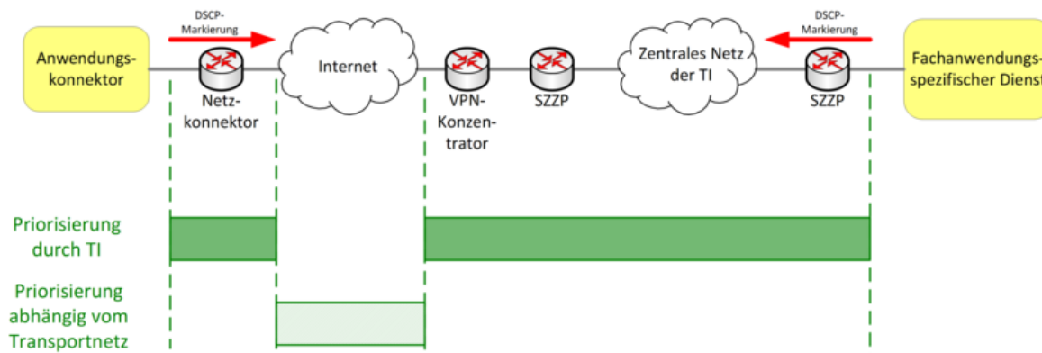
Abbildung 3: DSCP-Markierung (Beispiel)
