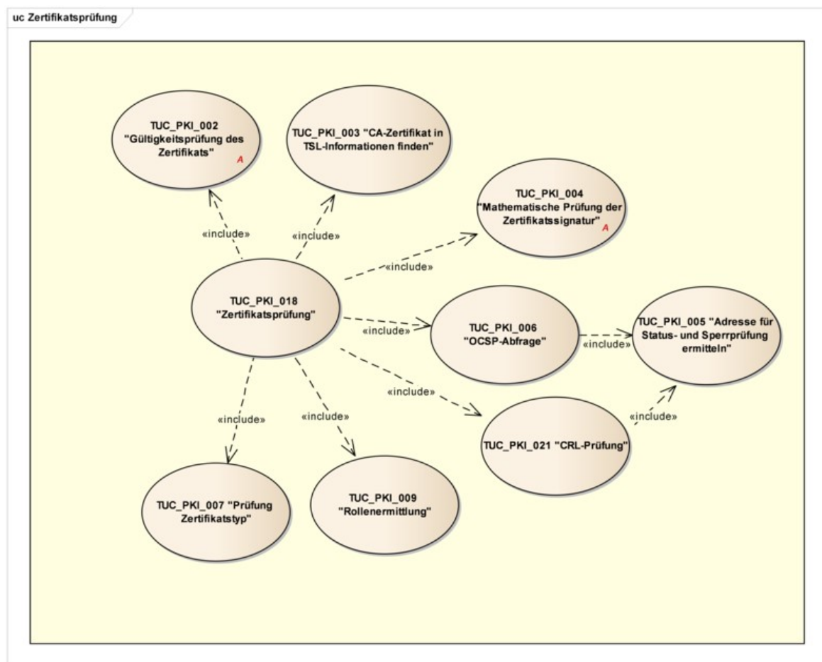
Abbildung 13: Use Case Diagram „Zertifikatsprüfung“
