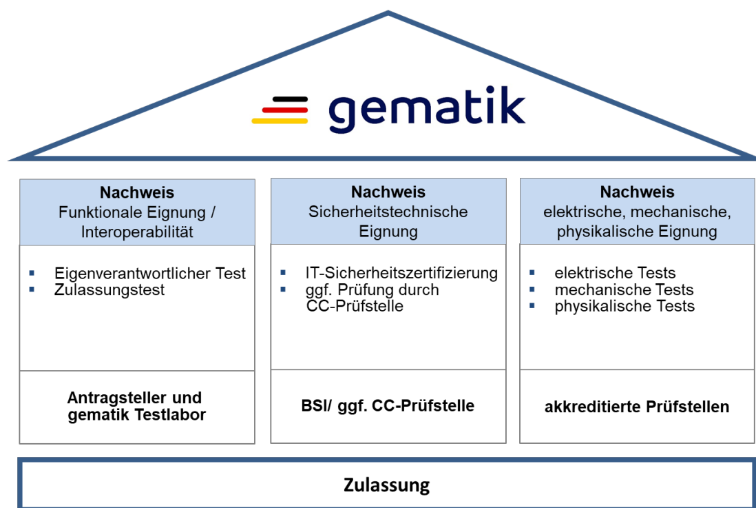
Abbildung 1: Prüfbereiche
