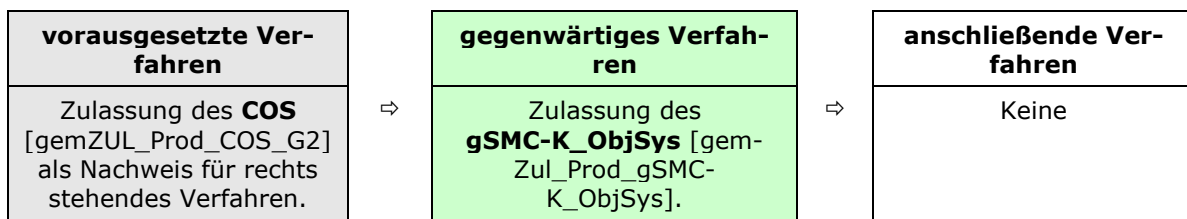
Abbildung 2: Reihenfolge Zulassungsverfahren
