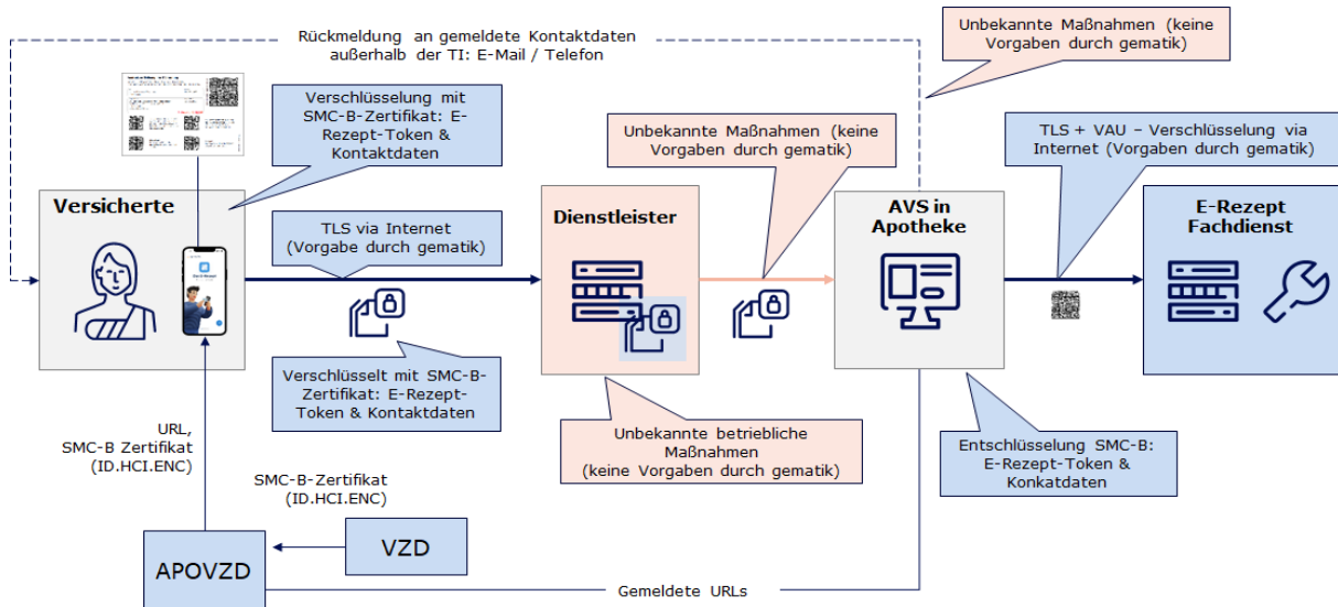
Abbildung 1: Schema Einlösen ohne Anmeldung am E-Rezept-Fachdienst im E-Rezept-FdV
