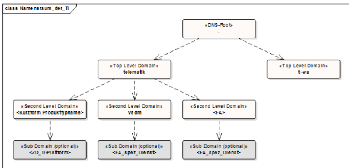
Abbildung 2: Domainnamen und hierarchische Struktur des Namensraums der TI
