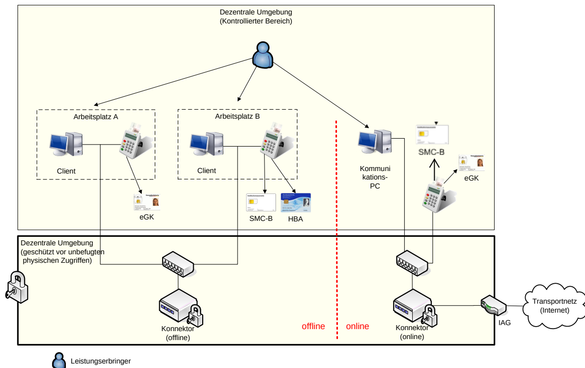
Abbildung 12: Standalone-Szenario mit physischer Trennung im Konnektor
